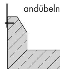
glatte Überfallkante
